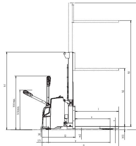
SBP12 / 14 / 16N3 ELEVACION INICIAL
