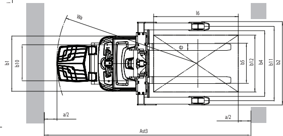
SBP16N3SR HORQUILLAS ANCHAS Y PLATAFORMA ABATIBLE
