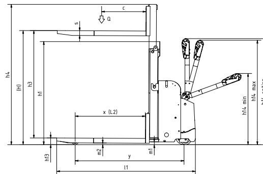
SBP12N2C APILADOR COMPACTO
