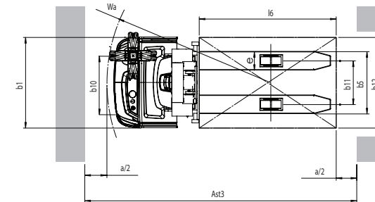
SBP12N2C APILADOR COMPACTO
